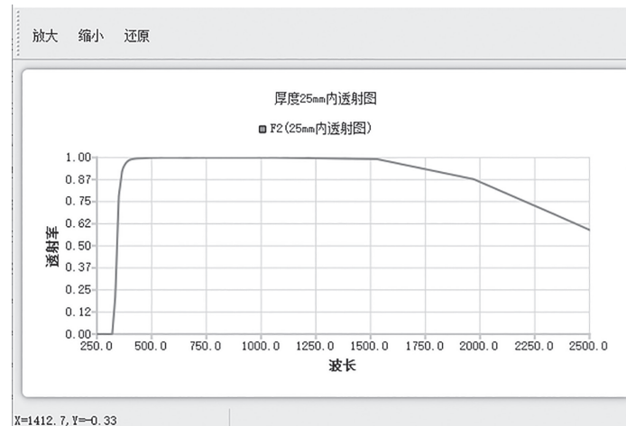
图 8 某一种型号的玻璃的内透射图
