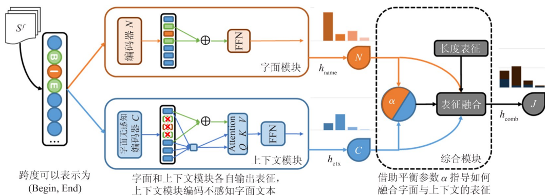
图1 NCMModel 模型网络结构
