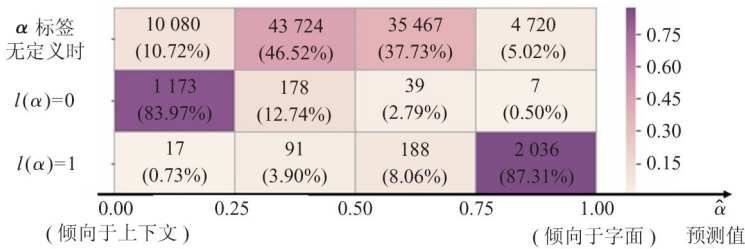
图 4 NCModel 模型中平衡参数的预测分布
